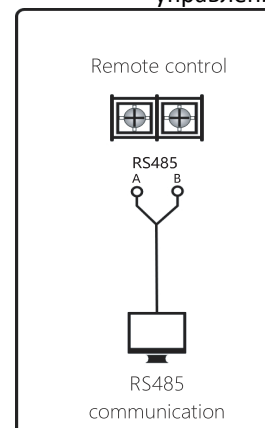
Подключение пульта управления
