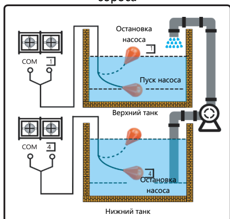
Подключение поплавковых выключателей для сброса
