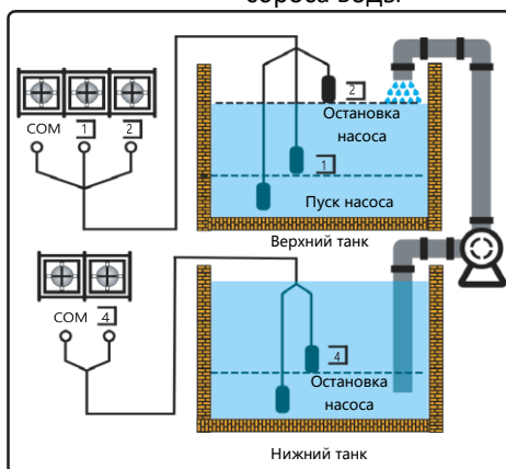
Подключение аналоговых датчиков для сброса воды
