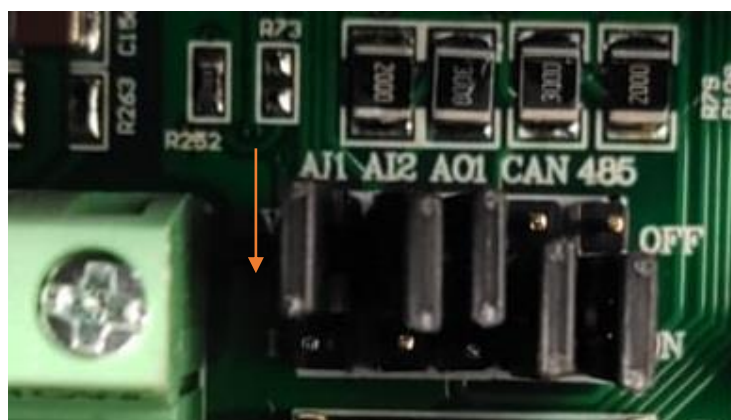
Рисунок 2. Установка перемычки входа AI1
