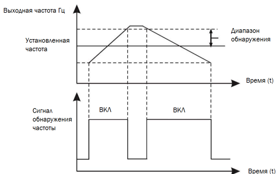
Рисунок 6-16 - Функция обнаружения заданной частоты
