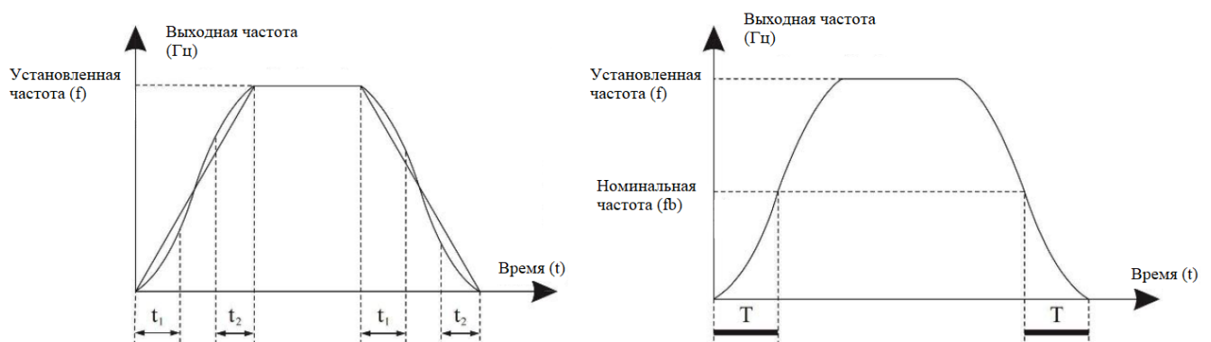
Рисунок 6-2 - S-образные кривые ускорения/замедления
