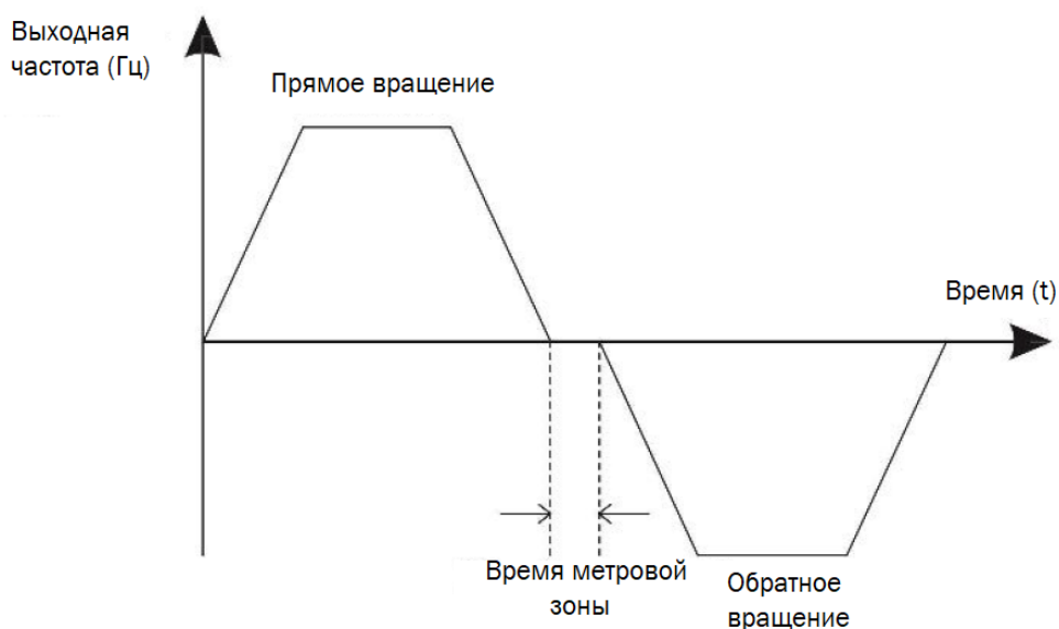
Рисунок 6-14 - Время мертвой зоны прямого/обратного вращения
