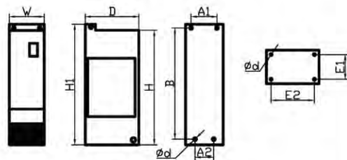
FD N 200-280 кВт
