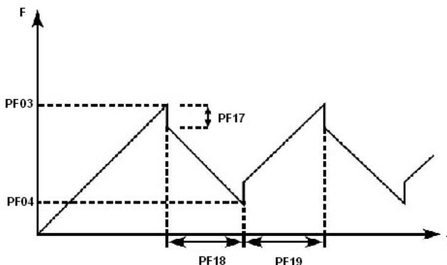
Параметры встроенного PID-регулятора
