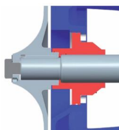
Двойное механическое уплотнение сифонного типа: Тип D – «спина к спине» Тип T – тандемное. M3+M3 или M7+M7
