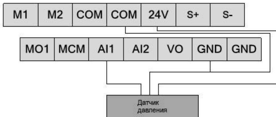
Схема подключения трехпроводного датчика давления
