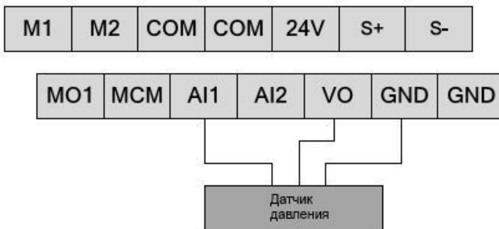
Схема подключения трехпроводного датчика давления
