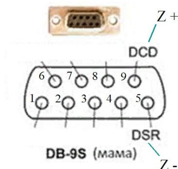
Рисунок 3. Схема подключения модуля связи
